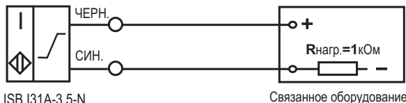
Схема подключения к оборудованию
